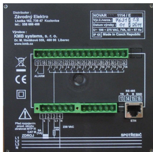
Obr. 2.6 : Zadní panel regulátoru s komunikačním rozhraním Ethernet
